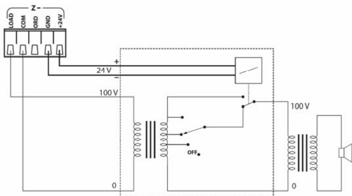
Sistema con Relè' di bypass 24V DC
