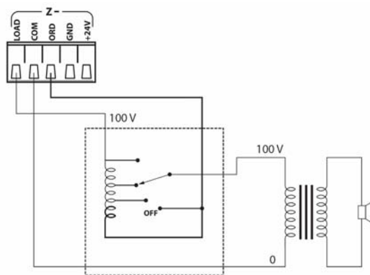
“3 Wires ” System
