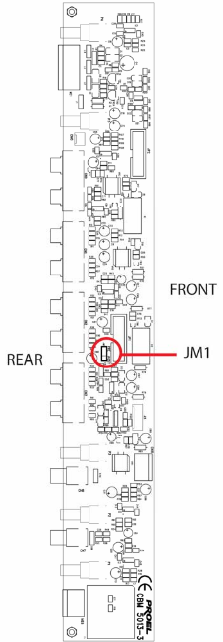
Scheda posteriore ingressi/uscite
