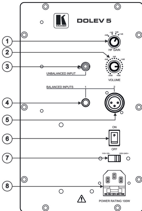
Рис. 1. Активная 2-полосная акустическая система студийного уровня с возможностью двойного усиления Dolev 5
