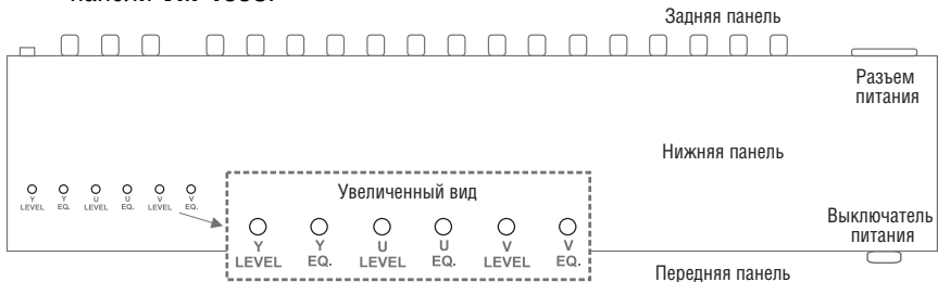
Рис. 2. Регуляторы на нижней стороне VM-100C
