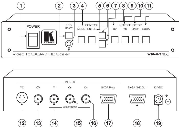
Рис. 1. Масштабатор VP-419xI (передняя и задняя панели)
