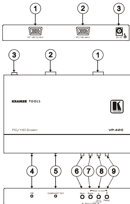
Рис. 1. Масштабор сигнала PC/HD VP-420 — органы управления и контроля
