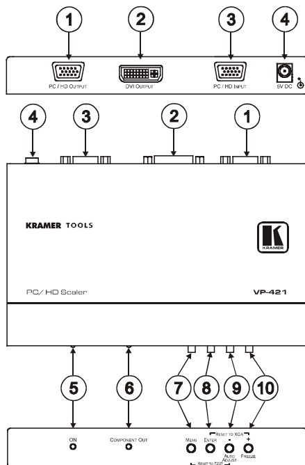
Рис. 2. Масштабор сигнала PC/HD VP-421— органы управления и контроля
