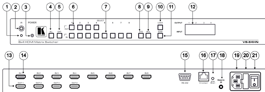
Рис. 1. Матричный коммутатор VS-84HN
