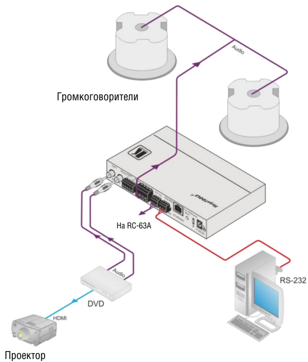
Рис. 1. Установка потолочного громкоговорителя закрытого типа Yarden 8-CN в зале заседаний
