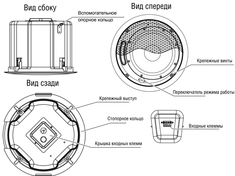
Рис. 2. Потолочный громкоговоритель закрытого типа Yarden 8-CH
