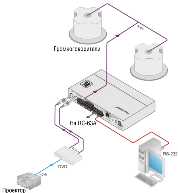
Рис. 1. Установка потолочного громкоговорителя закрытого типа Yarden 6-C в зале заседаний
