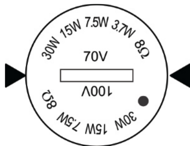
Рис. 7. Установка положения переключателя
