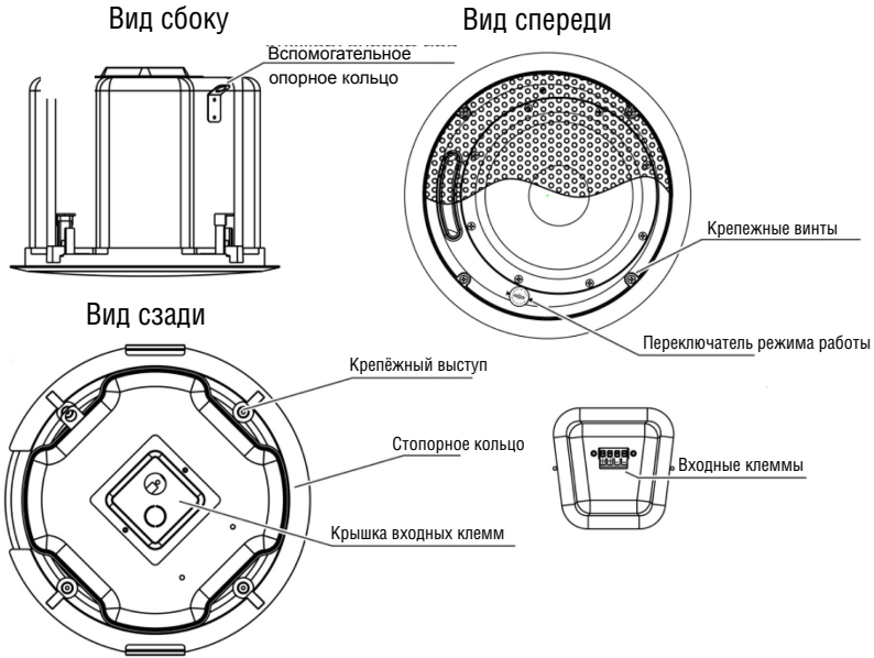
Рис. 2. Потолочный громкоговоритель закрытого типа Yarden 6-C
