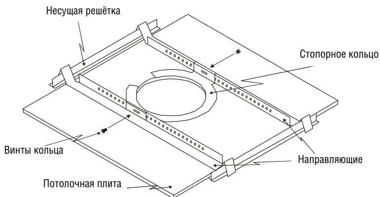
Рис. 4. Установка потолочного громкоговорителя закрытого типа Yarden 6-C
