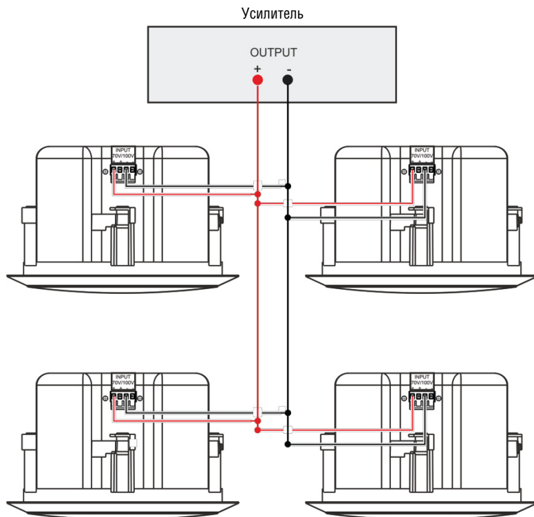
Рис. 10. Квадратная компоновка с параллельным подключением
